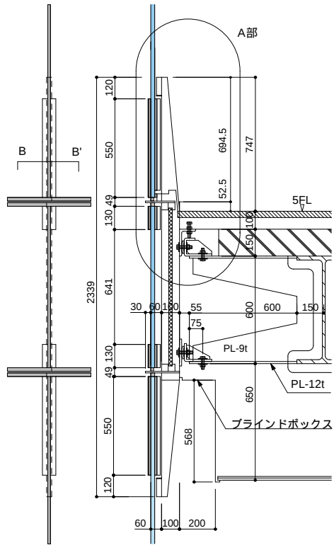
PFG構法立面図 S.1:30
