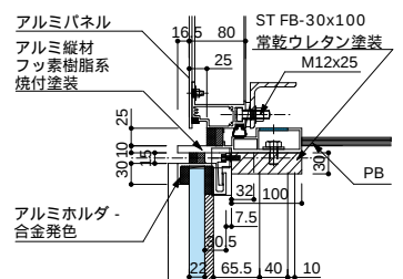
壁取り合い部平面詳細 S.1:12
