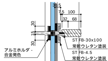
B-B'部詳細 S.1:12
