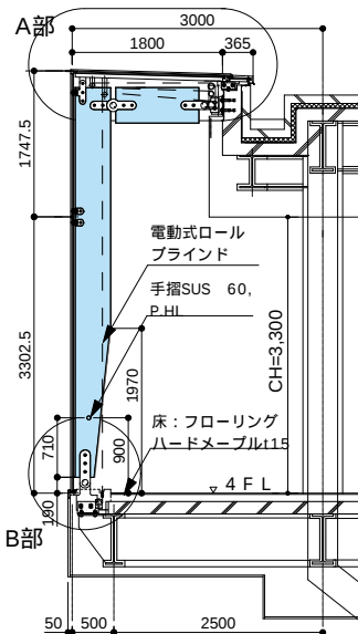
食堂開口部断面図 S.1:100
