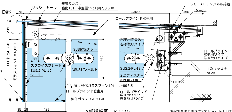
A部詳細図 S.1:20
