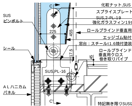
B部詳細図 S.1:20
