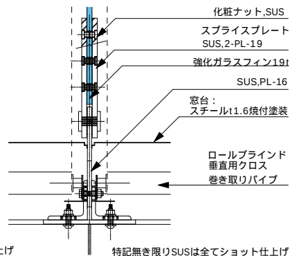
C-C'部詳細図 S.1:20
