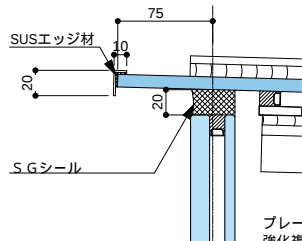
D部詳細図 S.1:6
