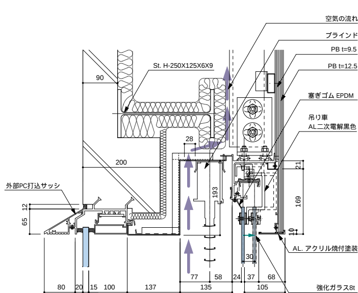
エアフローウィンド上部縦断面図 S.1:10
