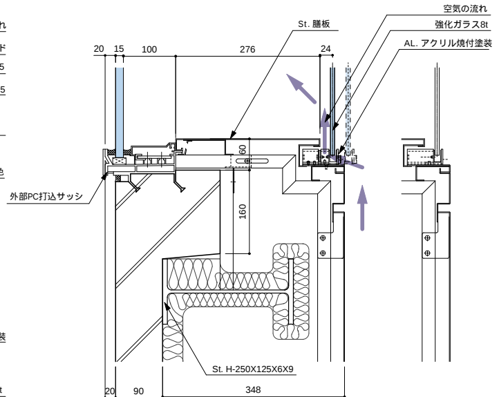
エアフローウィンド下部縦断面図 S.1:10
