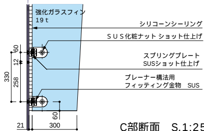
C部断面 S.1:25
