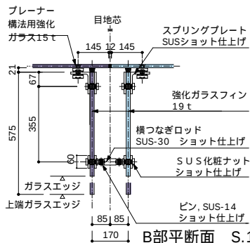
B部平断面 S.1:25
