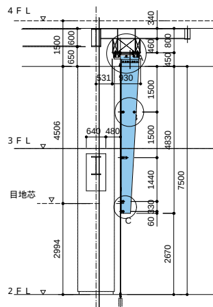
エントランス断面図 S.1:170
