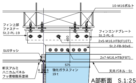
A部断面 S.1:25
