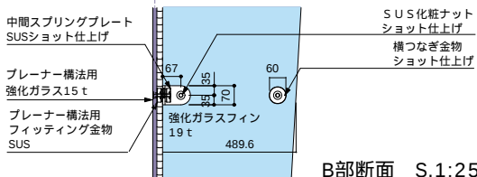
B部断面 S.1:25
