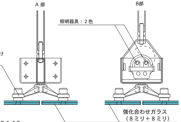
詳細図 S.1:10
