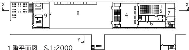
1階平面図 S.1:2000
