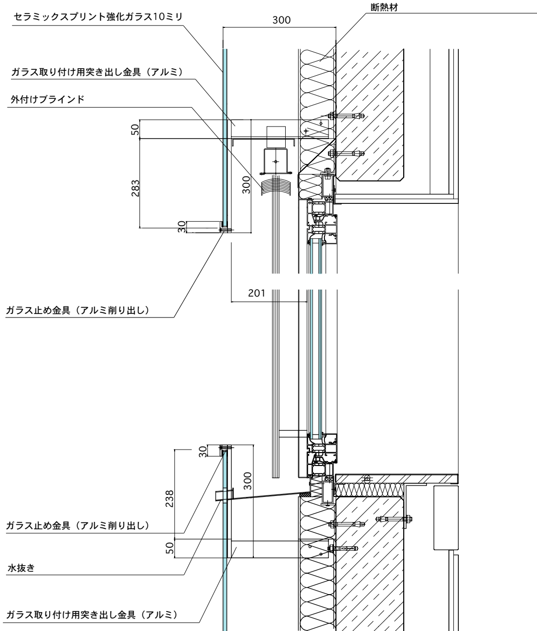
外壁・開口部詳細図 S.1:15
