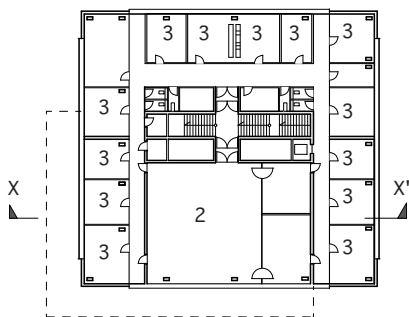
2階平面図 S.1:800
