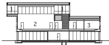
X-X'断面図 S.1:800
