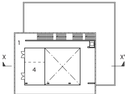
3階平面図 S.1:800
