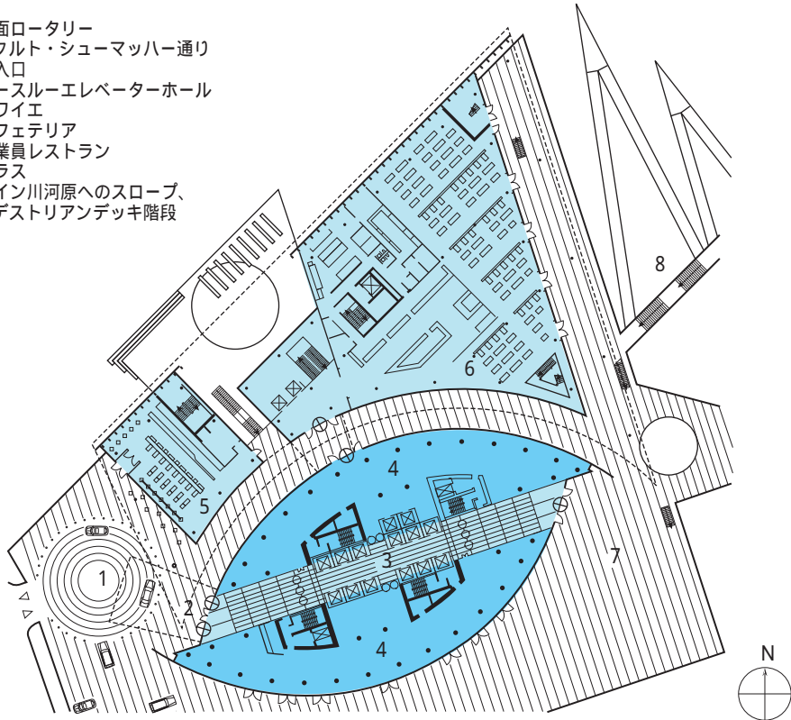
配置図・1階平面図 S.1:1200
