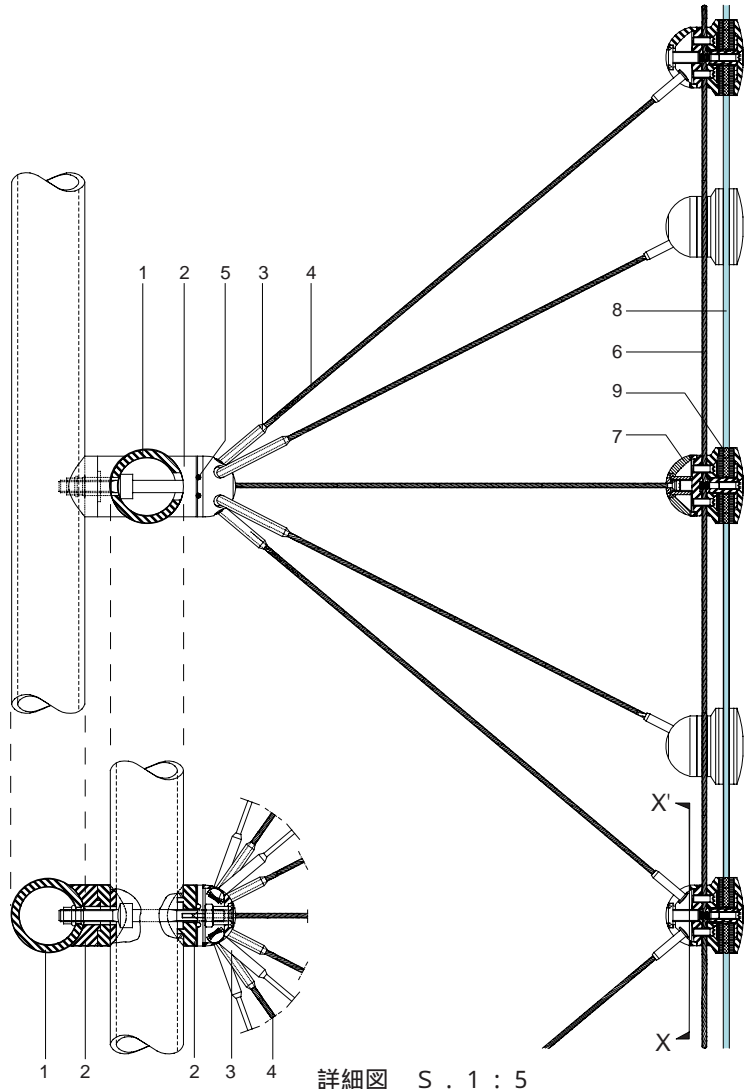
詳細図 S . 1 : 5
